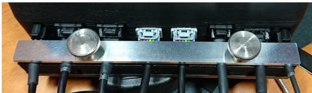
Led6 Afficheur pilote Alim. Capteur gauche Capteur Droit Boite à boutons GPS Répéteur audio
